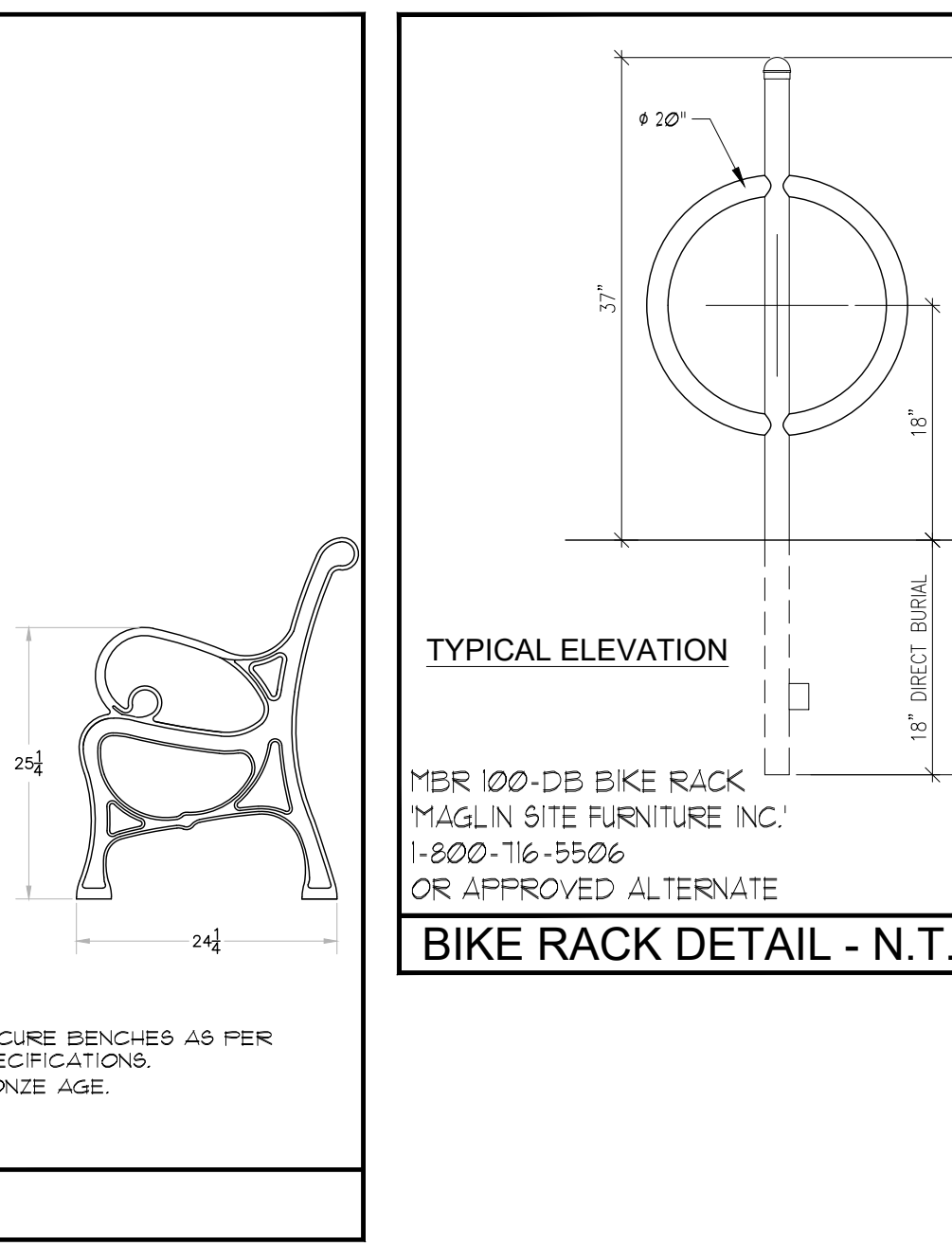
BIKE RACK DETAIL - N.T.S.
