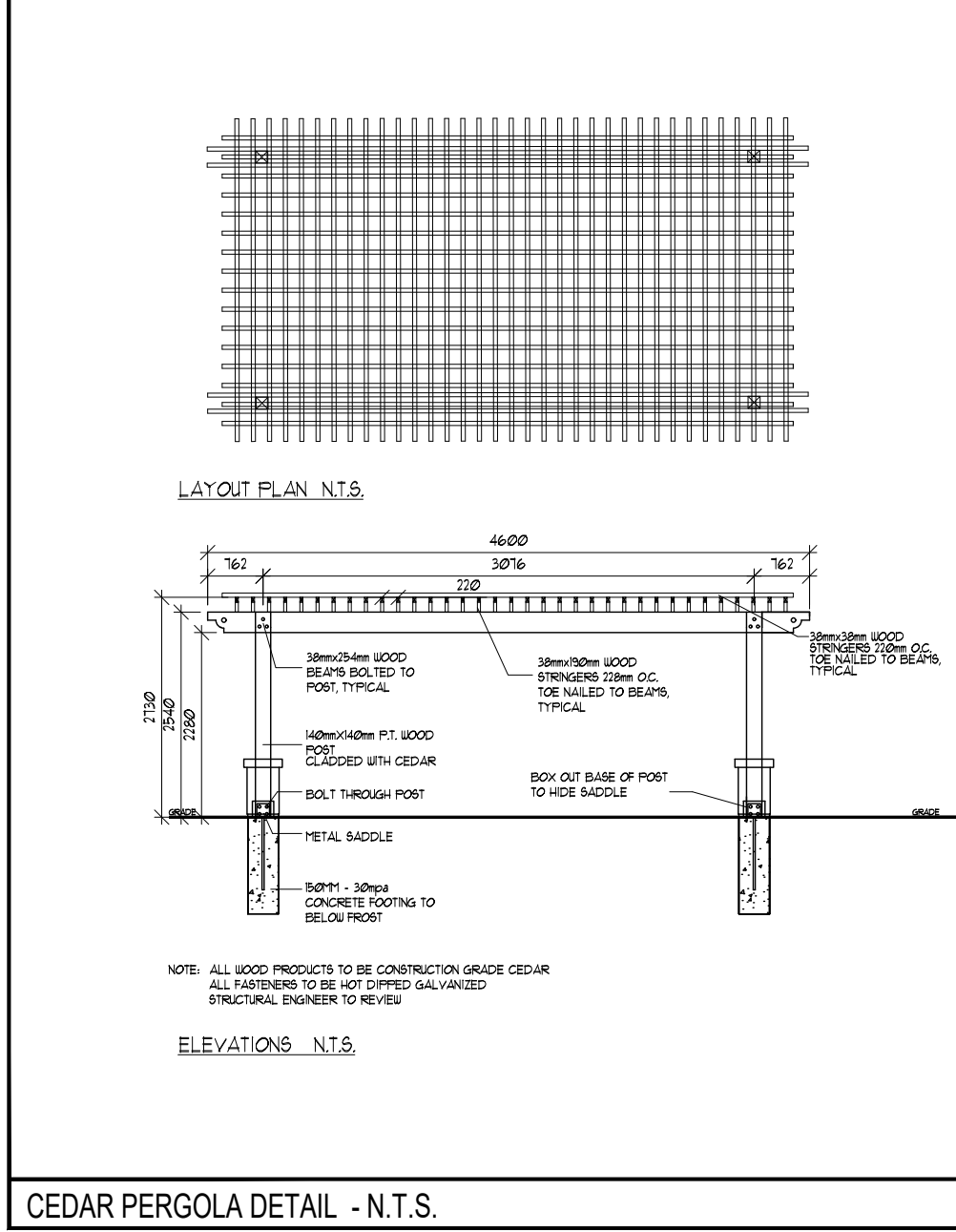
CEDAR PERGOLA DETAIL - N.T.S.
