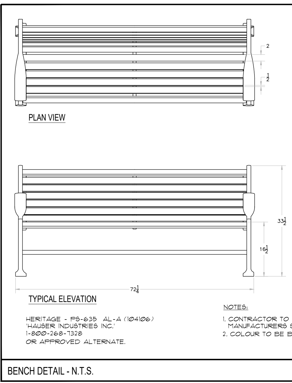
BENCH DETAIL - N.T.S.
